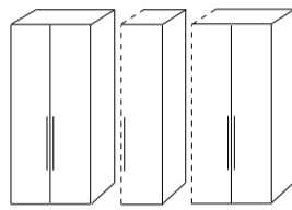
Türbreite/ door width: 50 cm 226 - 242(H) 40/ 60(T) 98/ 146/ 194/ 242/ 290 (B)
