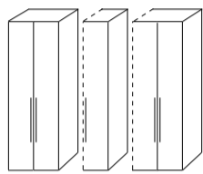
Türbreite/ door width: 38 cm 226 - 242(H) 40/ 60(T) 74/ 110/146/182/ 218 (B)
