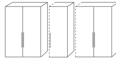
Türbreite/ door width: 74 cm 226 - 242(H) 40/ 60(T) 146/ 218/ 290/ 362/ 434 (B)
