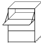
2 Schubkästen / 1 Klappfach 2 drawers / 1 flap 69/88(B) 109,8(H)
